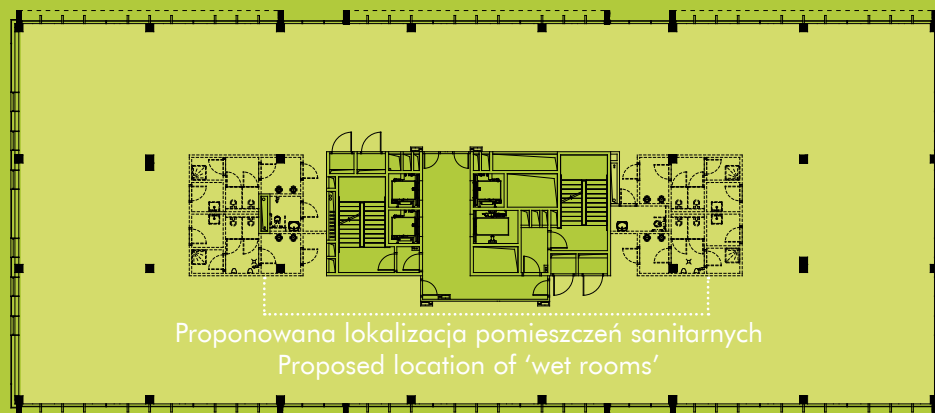
Rzut typowego piętra Standard floor plan
