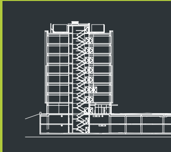
Przekrój Cross section
